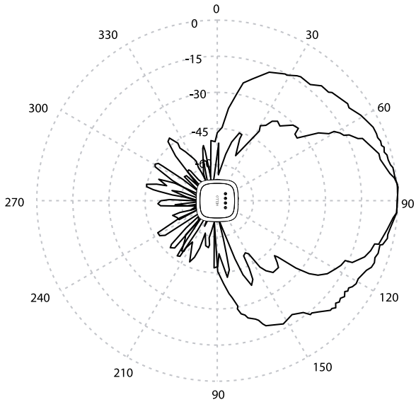
Alcance de vigilancia por radar.
